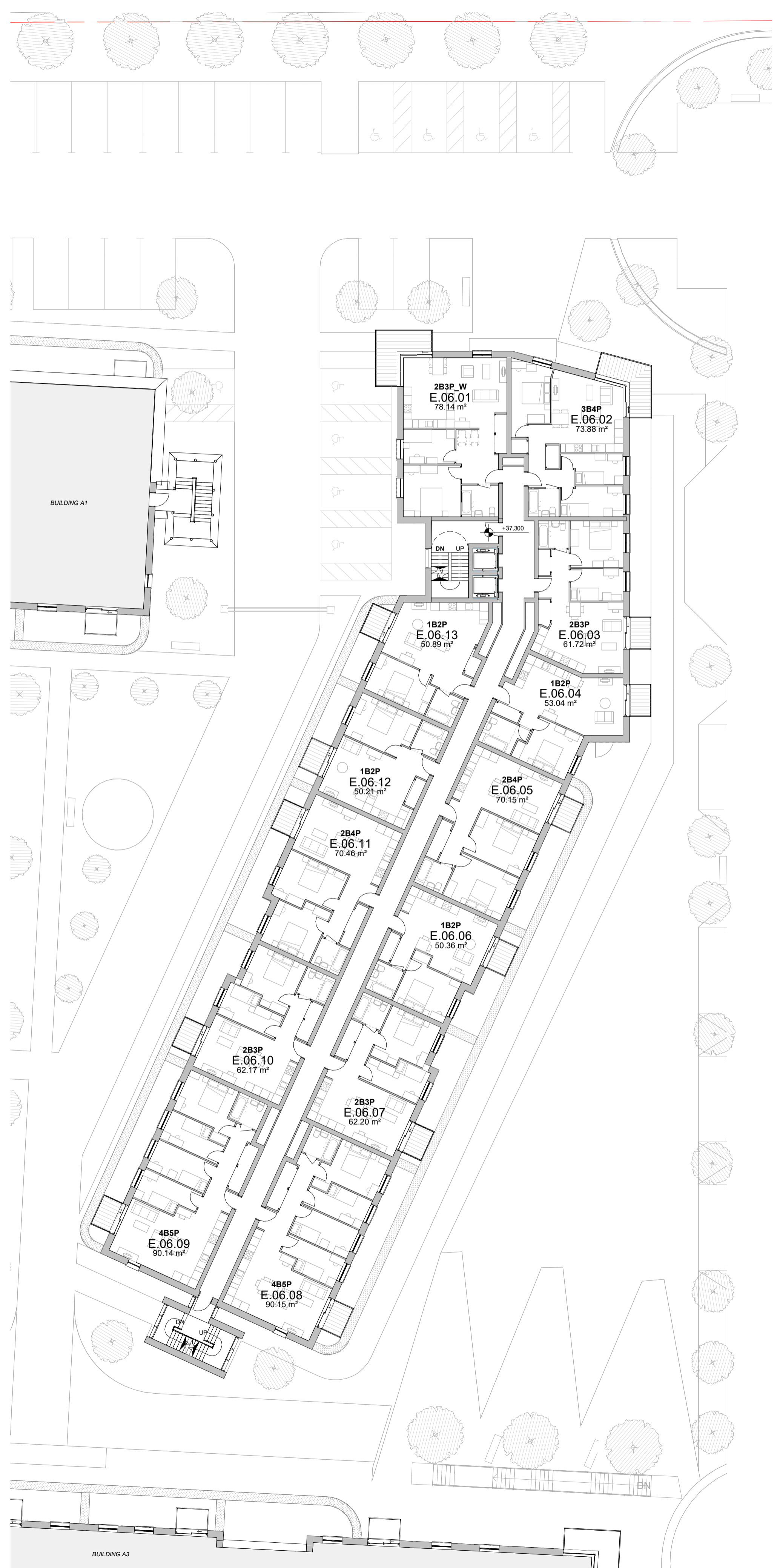
2 Level 6 +37.300 AOD 1:200
